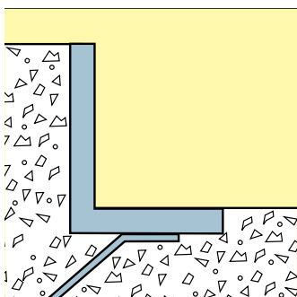
Kåbe 25R. Til måtter og gitre med en højde på 25 mm. Profil 31 x 25 x 4 mm.
