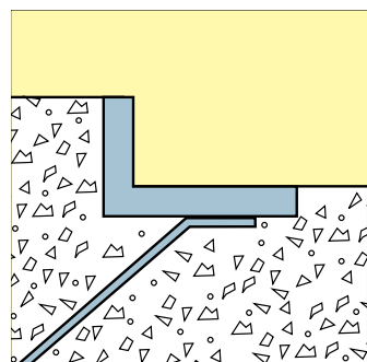
Kåbe 12R. Til måtter med en højde på 10-14 mm. Profil 16 x 26 x 4 mm.
