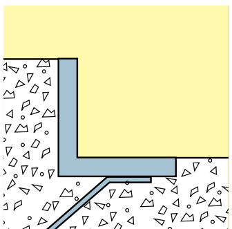
Kåbe 22R. Til måtter og gitre med en højde på 20-22 mm. Profil 25 x 25 x 3 mm.
