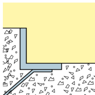
Kåbe 17R. Til måtter og gitre med en højde på 15-20 mm. Profil 20 x 30 x 3 mm.
