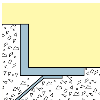
Kåbe 20R. Til måtter og gitre med en højde på 20-22 mm. Profil 25 x 31 x 4 mm.
