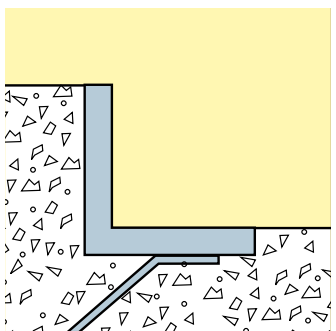
Kåbe 22R. For matter og rister høyde 20-22 mm. Profil 25 x 25 x 3 mm.
