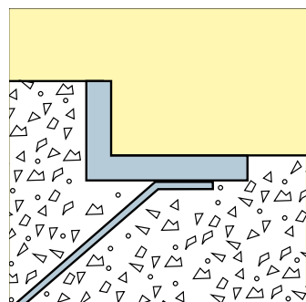
Kåbe 12R. For matter høyde 10-14 mm. Profil 16 x 26 x 4 mm.
