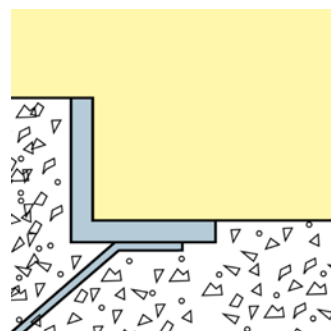
Kåbe 17R. For matter og rister høyde 15-20 mm. Profil 20 x 30 x 3 mm.
